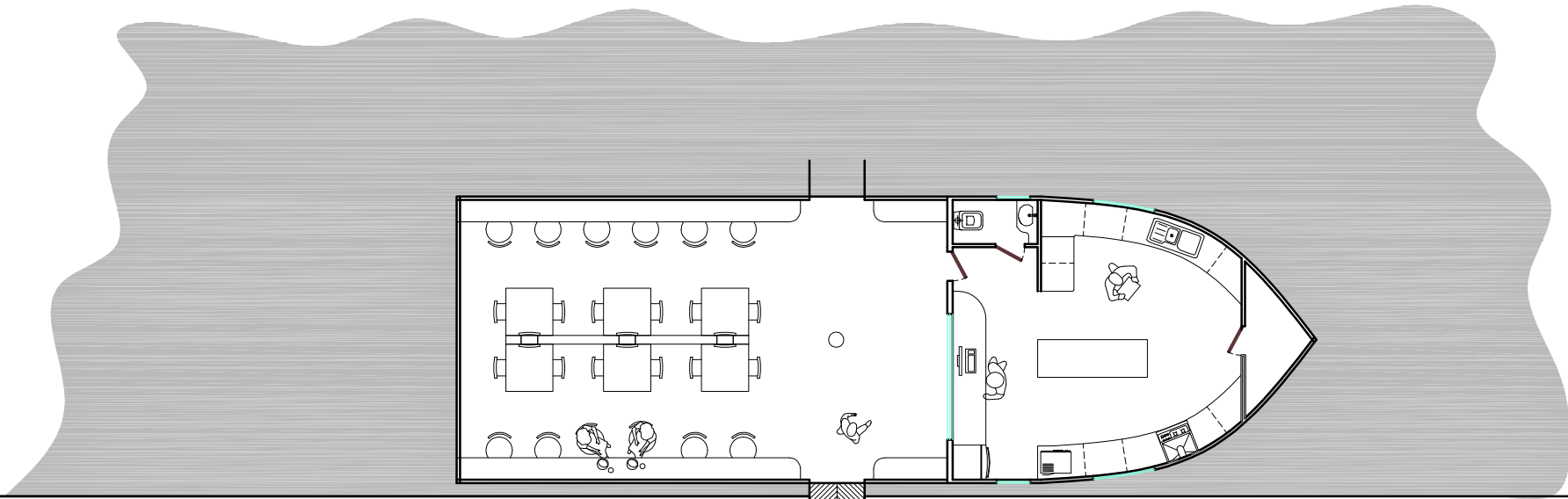
Progetto per PUB da realizzarsi su barca
