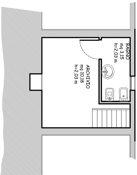
PIANO INTERRATO stato precedente
