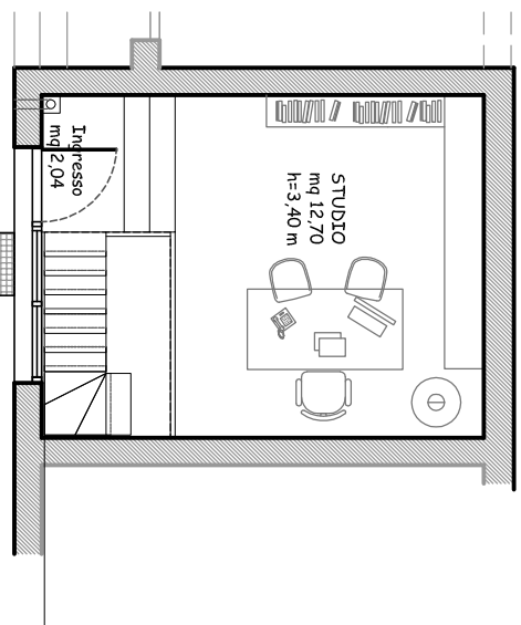
PIANO TERRA stato realizzato
